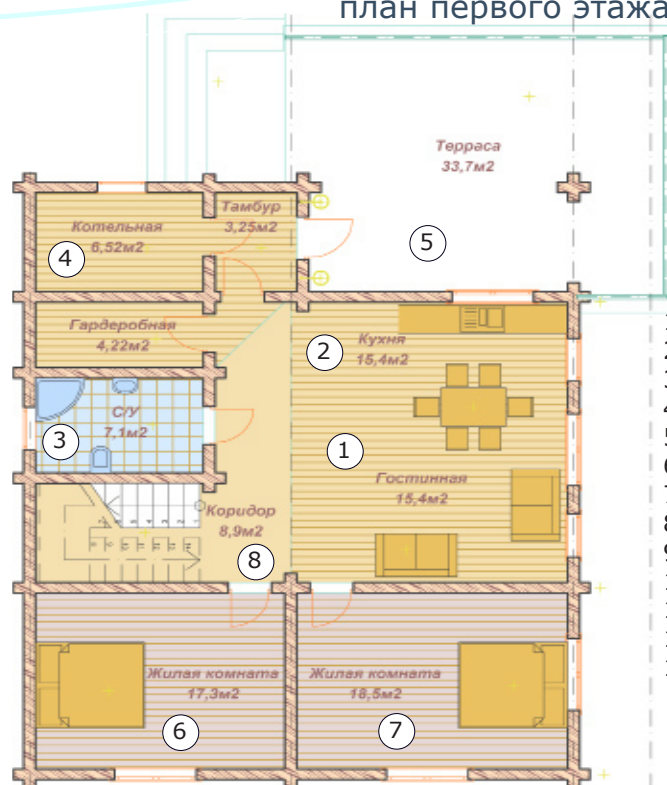
план первого этажа
